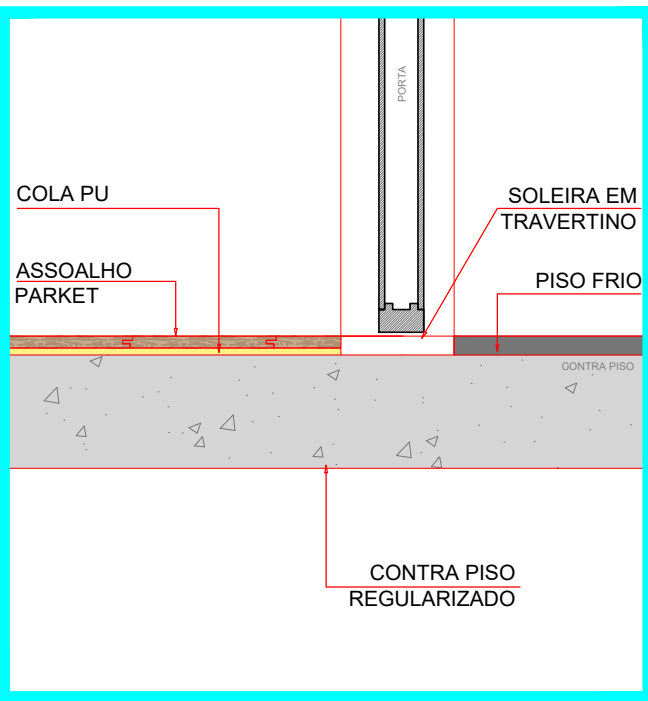
DET. 04 - TRANSIÇÃO DE PISO 1:10
