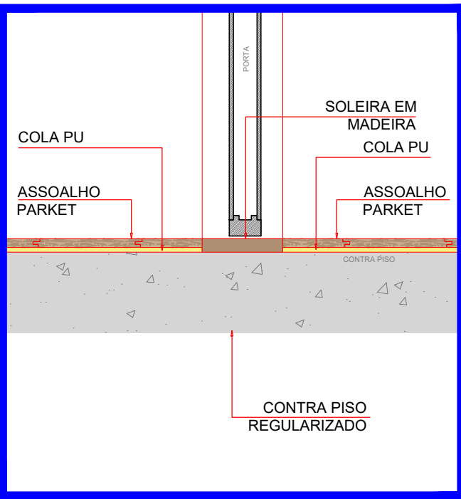
DET. 02 - TRANSIÇÃO DE PISO 1:10
