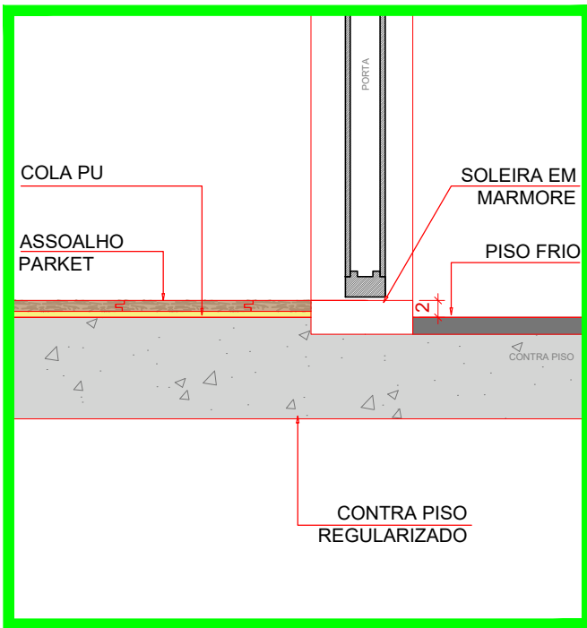
DET. 03 - TRANSIÇÃO DE PISO 1:10
