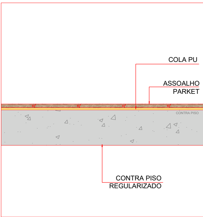
DET. FIXAÇÃO DE ASSOALHO 1:10
