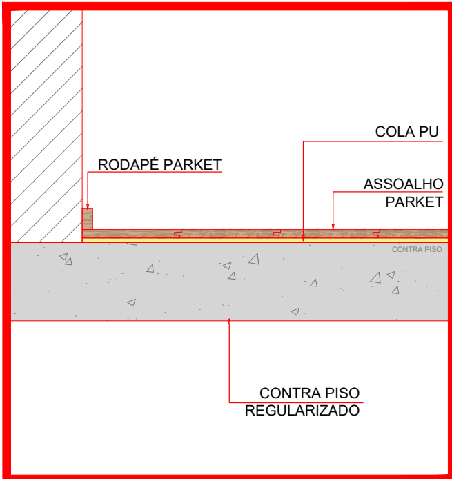
DET. 01 - RODAPÉ 1:10
